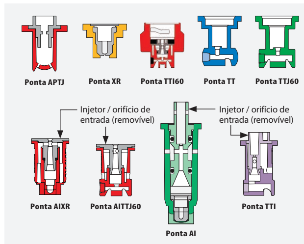
Figura 4. Desenho de corte de seções das pontas de pulverização APTJ, XR, TT, TTJ60, AIXR, AITTJ60, AI, TT160.
