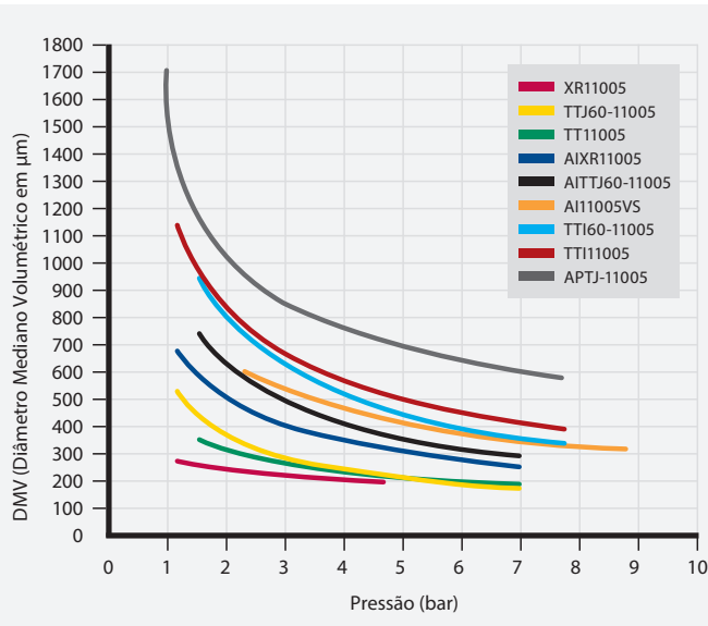
Figura 3. Diâmetros volumétricos de gotas das pontas de pulverização XR, TT, TTJ60, AIXR, AI, AITTJ60, TT160, TTI e APTJ em relação à pressão.
